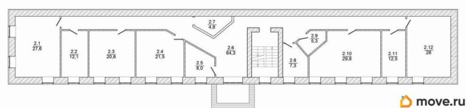
План 2 этажа
